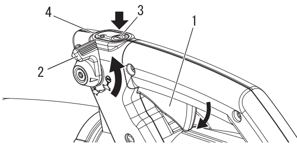
1. Interrupteur à poussoir 2. Levier de commande de vitesse 3. Bouton d'alimentation 4. DEL du témoin d'alimentation
